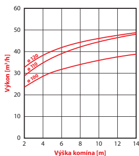
Nákres výkonu komínových nástavcov airhawk CILINDER ø 100, 110, 120 mm v závislosti na výške komína pri nulovej rýchlosti vetra.
