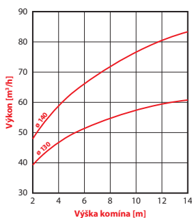
Nákres výkonu komínových nástavcov airhawk CILINDER ø 130, 140 mm v závislosti na výške komína pri nulovej rýchlosti vetra
