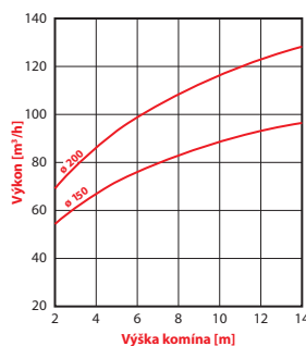
Nákres výkonu komínových nástavcov airhawk CILINDER ø 150, 200 mm v závislosti na výške komína pri nulovej rýchlosti vetra
